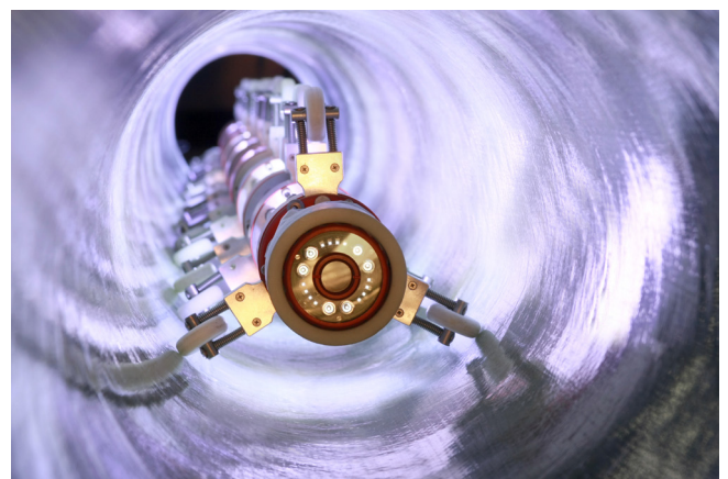
UV-Lichtquelle im Berolina-Liner (DN 300)
